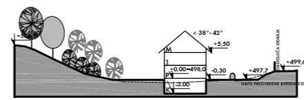
PREREZ B-B'
