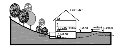
PREREZ C-C'
