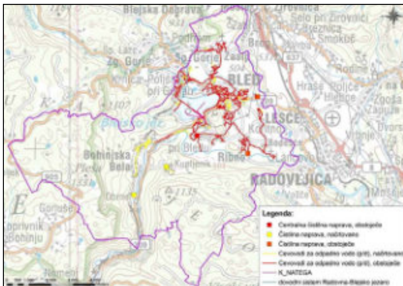
Slika 2-6: Kanalizacijski sistem v občini Bled
