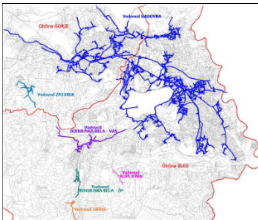
Slika 3-3: Shematski prikaz vodovodov v občini Bled (vir: Letno poročilo, Infrastrukture Bled d.o.o., februar 2012)
