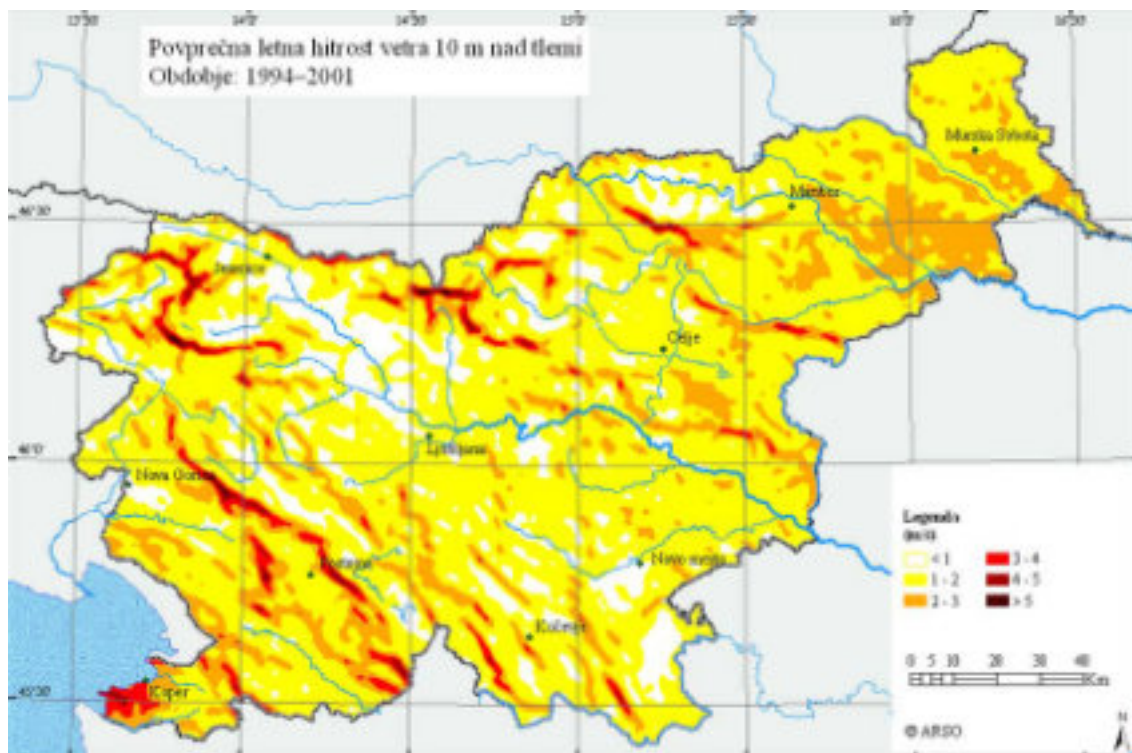
Slika 1-2: Povprečna letna hitrost vetra v višini 10 m od tal v letih 1994-2001 (vir: ARSO)
