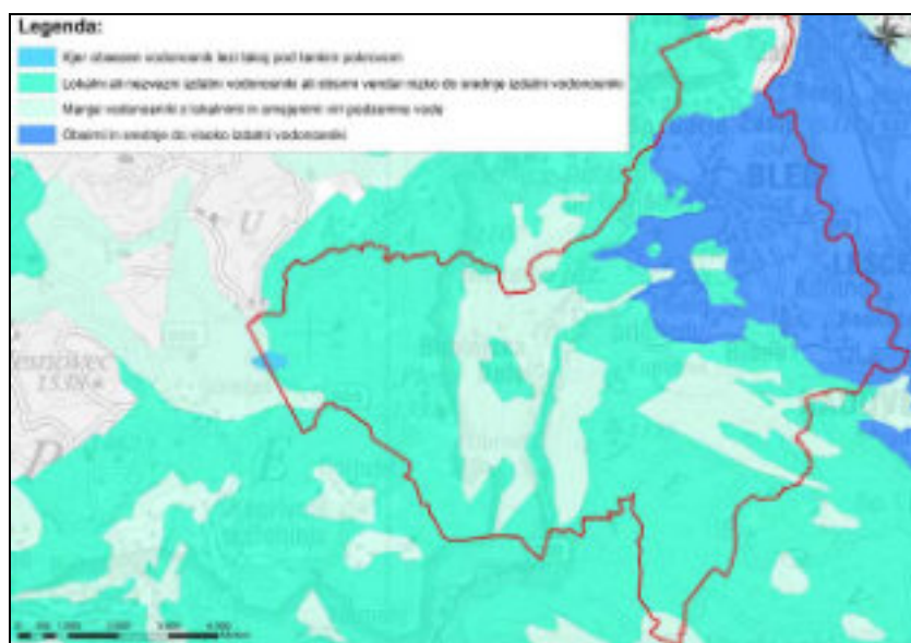
Slika 2-11: Hidrogeološka karta po IAH (vir: MKO-ARSO)
