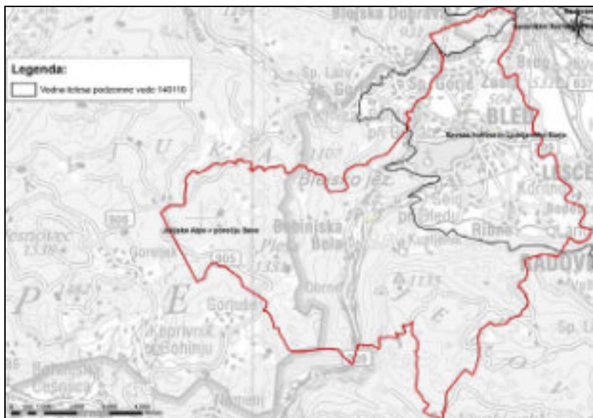
Slika 2-12: Vodna telesa podzemne vode (vir: MKO-ARSO)
