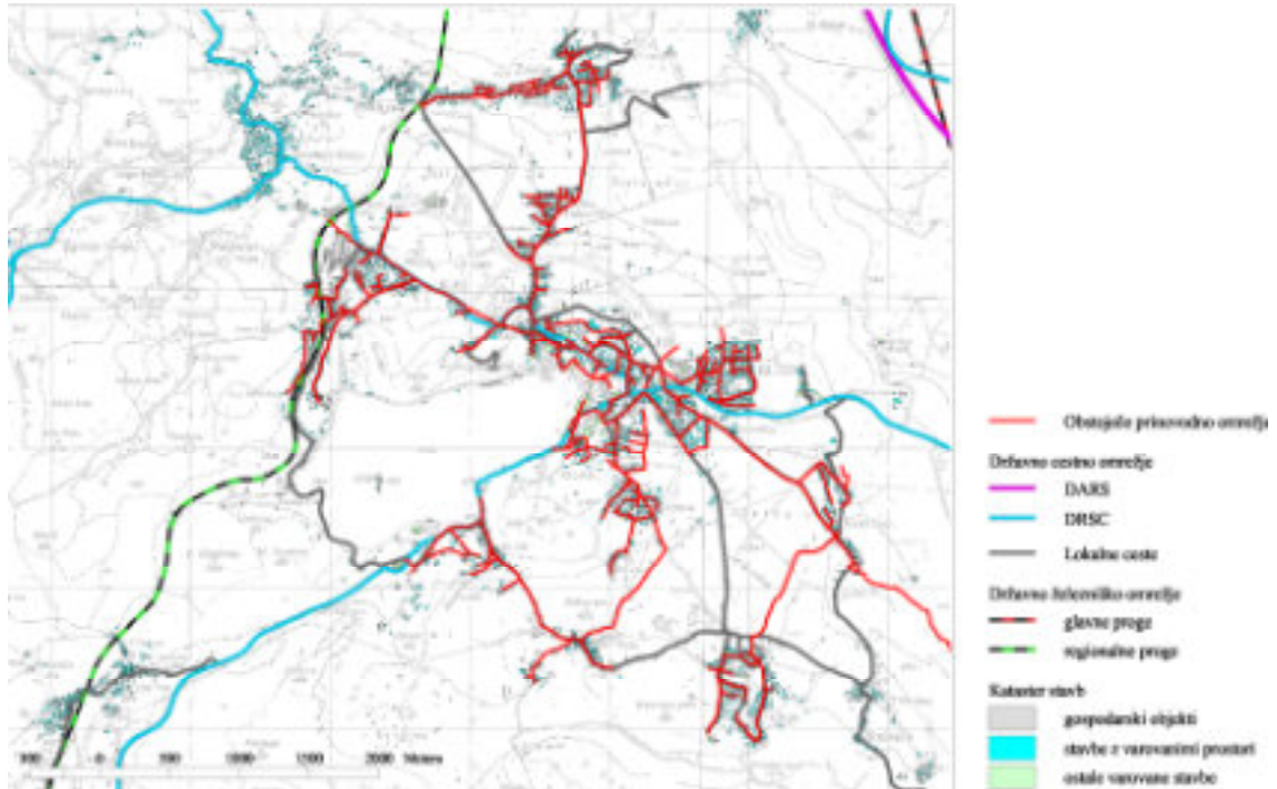
Slika 1-4: Omrežje zemeljskega plina v občini Bled – stanje 2012
