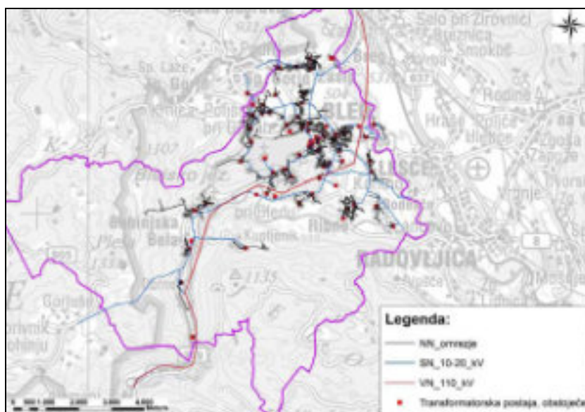
Slika 5-1: Obstoječe elektro omrežje in objekti v občini Bled
