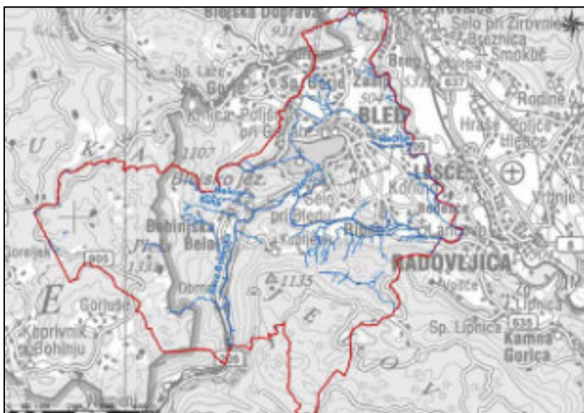
Slika 2-2: Rečna mreža na območju občine Bled
