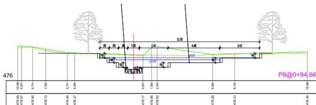
Slika: Terasasti profil za posedanje
