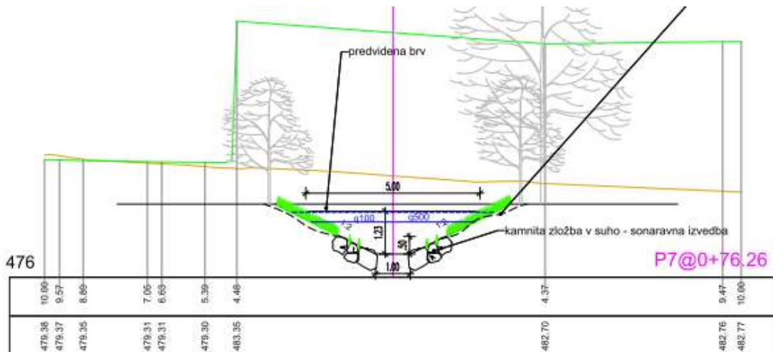
Slika: Struga neposredno gorvodno od Kidričeve ceste
